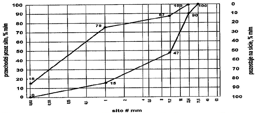
Rys. 4. Krzywe graniczne uziarnienia mieszanki kruszyw 0/22,4 mm do górnej warstwy podłoża ulepszonego
