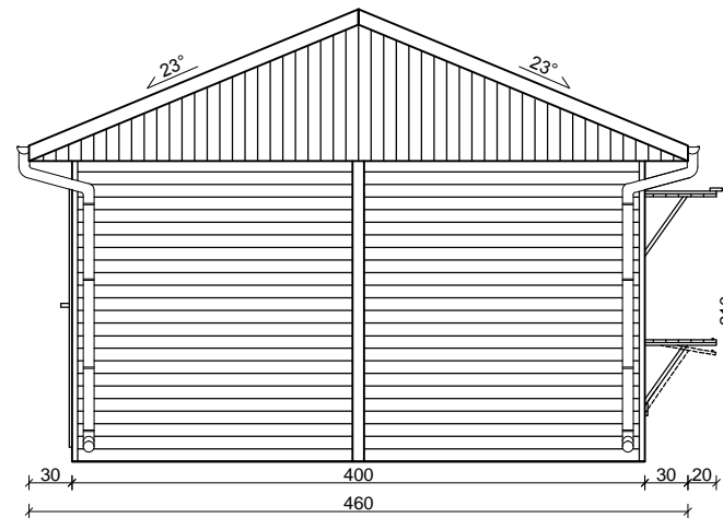
ELEWACJA TYLNA
