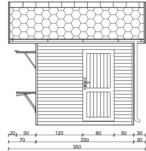
ELEWACJA BOCZNA
