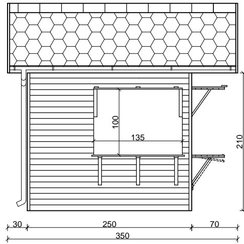
ELEWACJA BOCZNA
