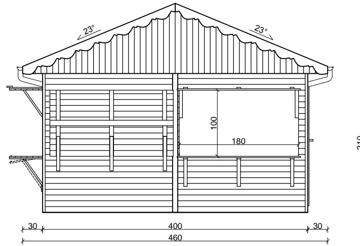
ELEWACJA TYLNA
