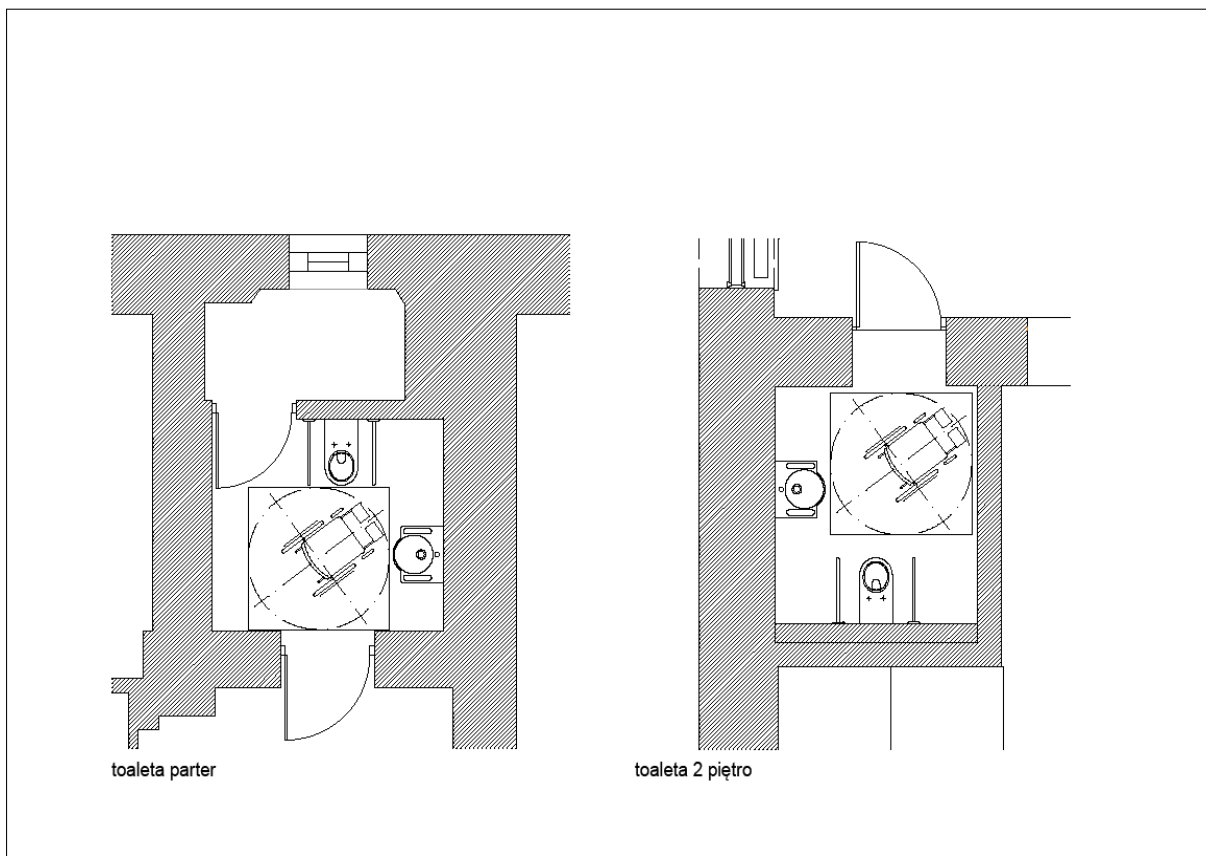
Rys. 2. Rzuty toalet (opracowanie ARCHIGRAF)
