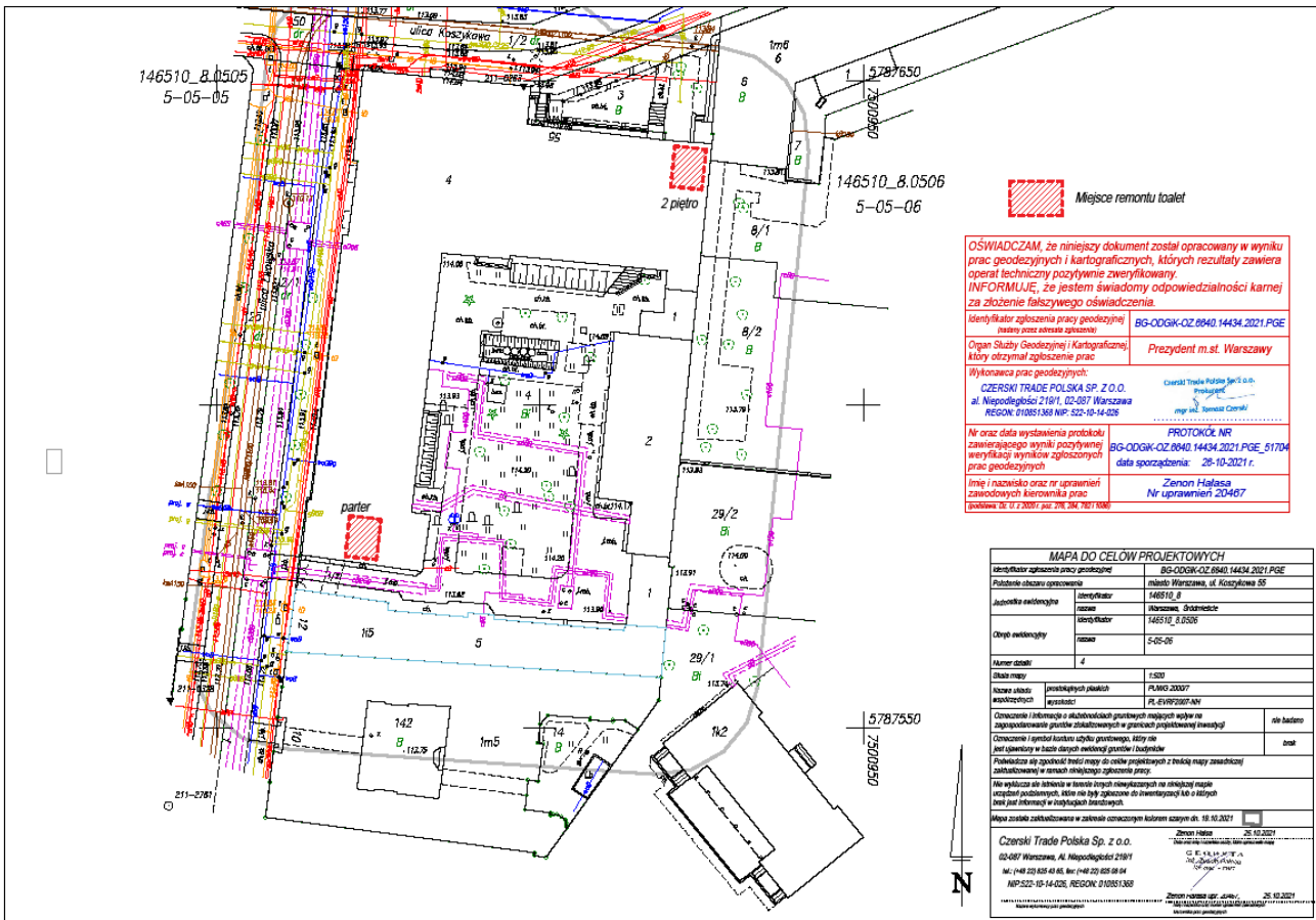
Rys. 1. Miejsce remontu toalet (opracowanie ARCHIGRAF)
