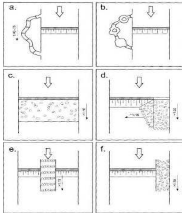
Rys. 6. Schematy współczesnych przejść dla ryb (Mokwa i Wiśniewski 2008)
