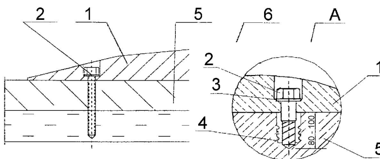
Rys. 4. Przykład umocowania progów do nawierzchni jezdni
