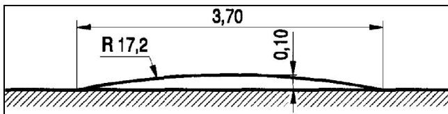
3.2. Próg płytowy z powierzchniami najazdowymi łukowymi (U-16b)
