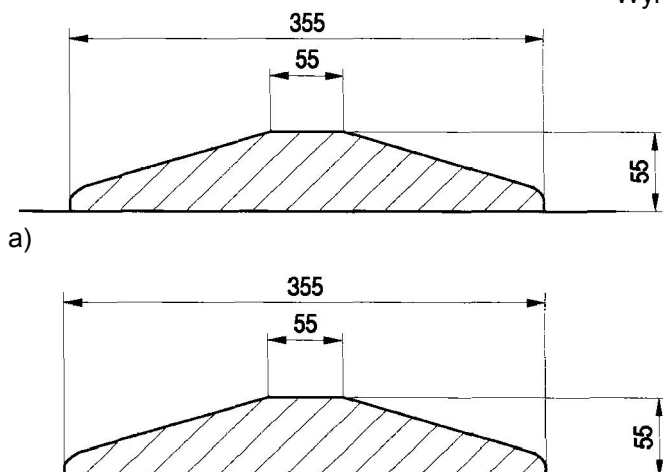
KSZTAŁT I WYMIARY W PRZEKROJU POPRZECZNYM PRZYKŁADOWYCH PROGÓW PODRZUTOWYCH (wg [23]) Wymiary w mm
